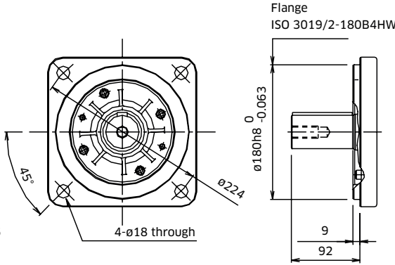
ISO Type
