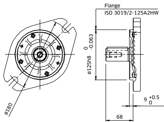
ISO Type
